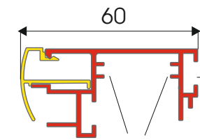
Eckverbinder Aluminium EV-A K60 wird in Nut eingeschoben und mit Inbusschrauben gesichert
