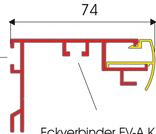
Eckverbinder EV-A K74 wird mit Schrauben gesichert
