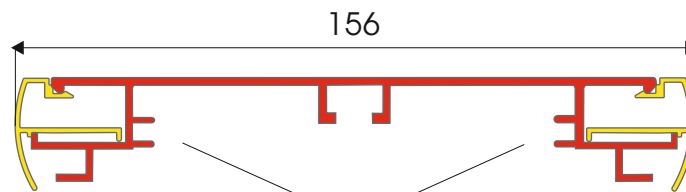
Eckverbinder EV-A K156 wird in Nut eingeschoben und mit Schrauben gesichert
